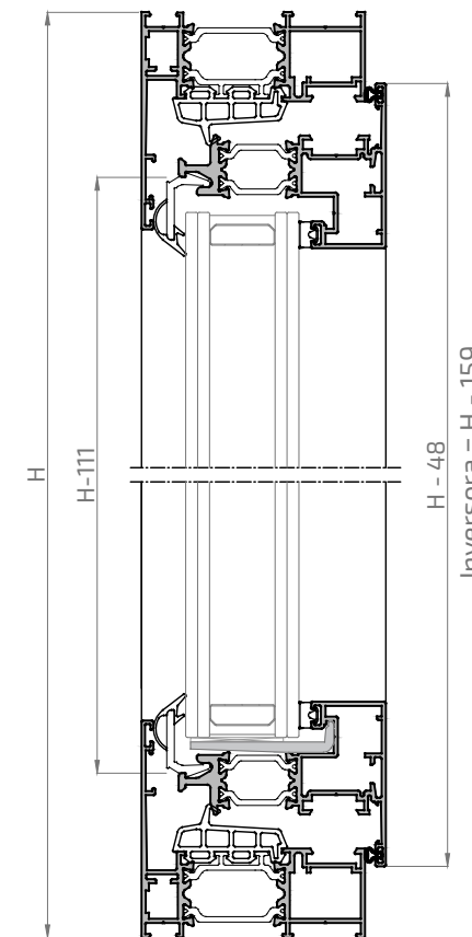
Sección B-B'
