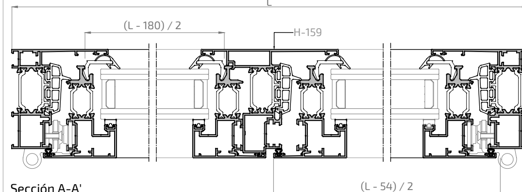
Sección A-A'
