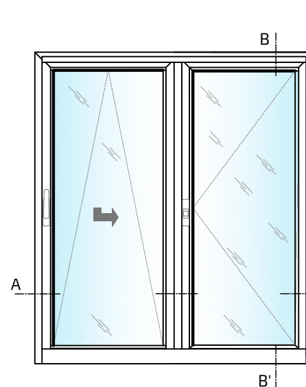
Sección B-B'
