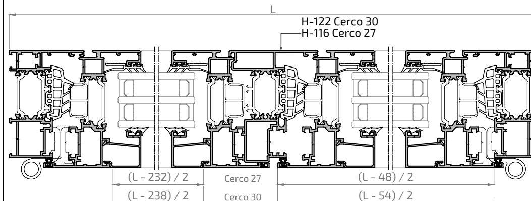
Sección A-A'
