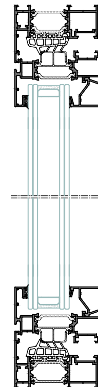
Sección B-B'
