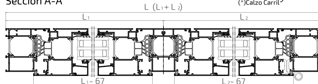
Sección A-A'
