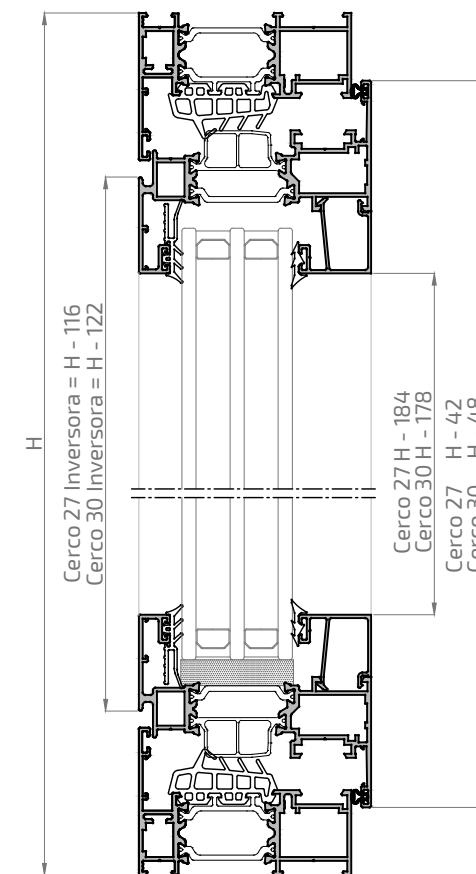
Sección B-B'
