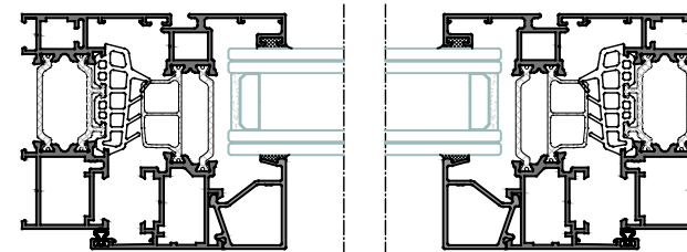
Sección A-A'
