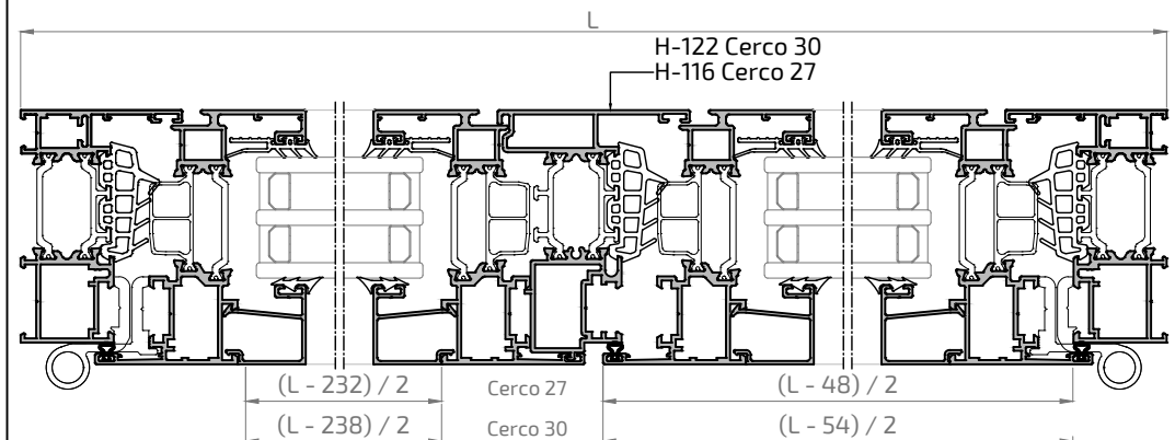
Sección A-A'
