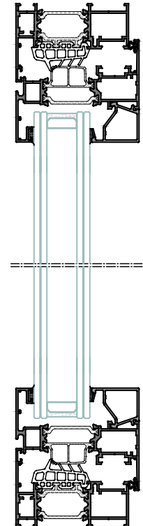
Sección B-B'
