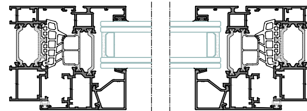
Sección A-A'
