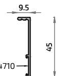
16322 Solapa clip 45 mm
