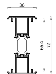
8482L Unión de Cercos alg 65
