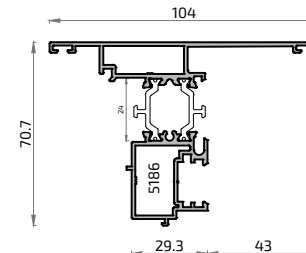
16766L Acople Inversora ALG 65 HS
