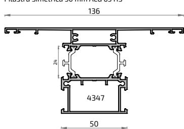
16768L Pilastra Simétrica 50 mm ALG 65 HS
