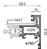
21428L Hoja Alg 65 Acrist. 43 mm
