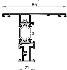
20560L Pilastra reducida hoja oculta
