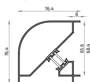
10006M Esquinero 90° Curvo
