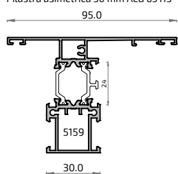
16767L Pilastra asimétrica 30 mm ALG 65 HS
