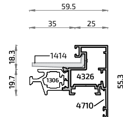
20223L Hoja ALG 65 HS
