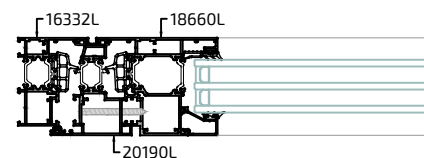
Sección A-A'
