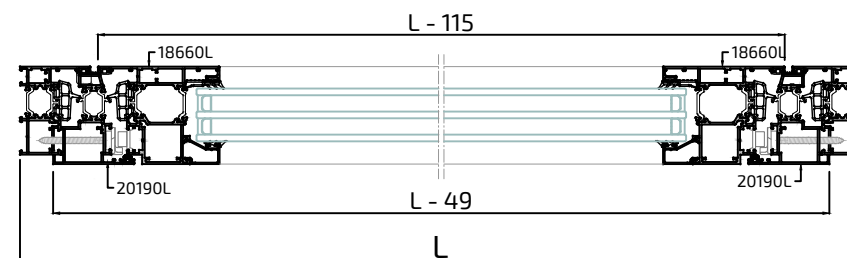
Sección B-B'
