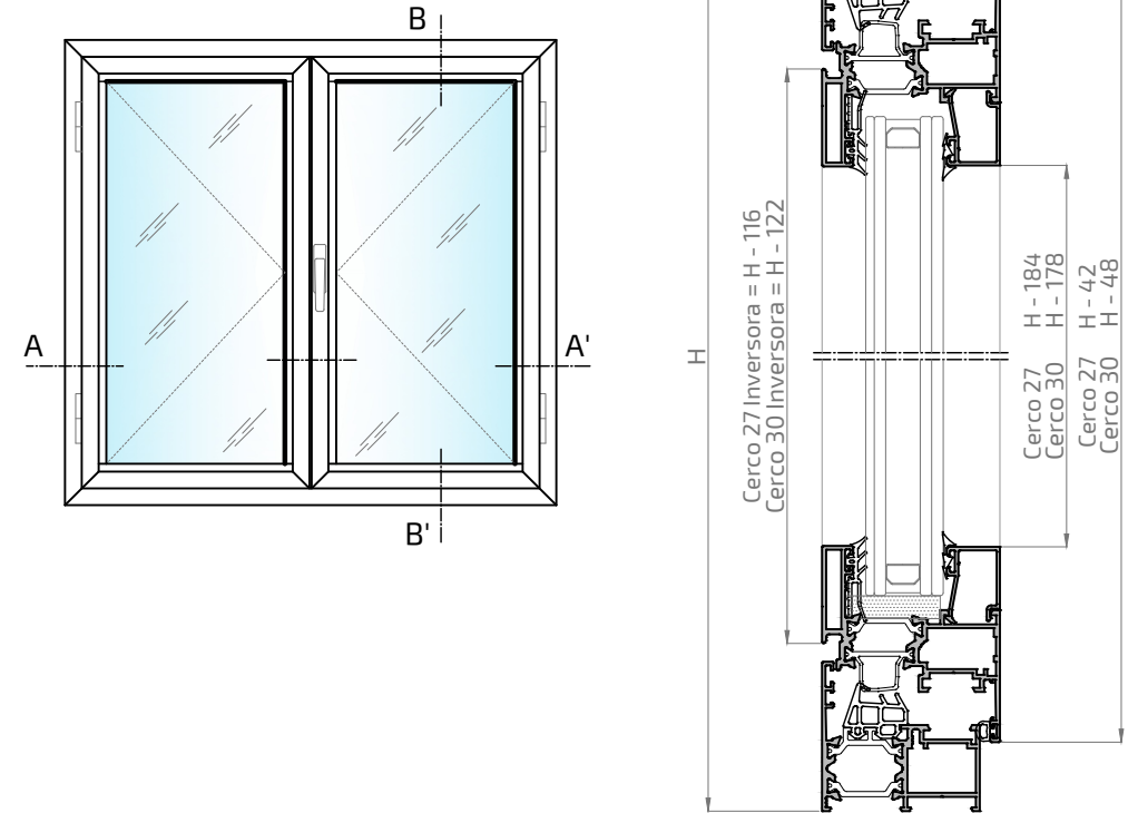
Sección B-B'
