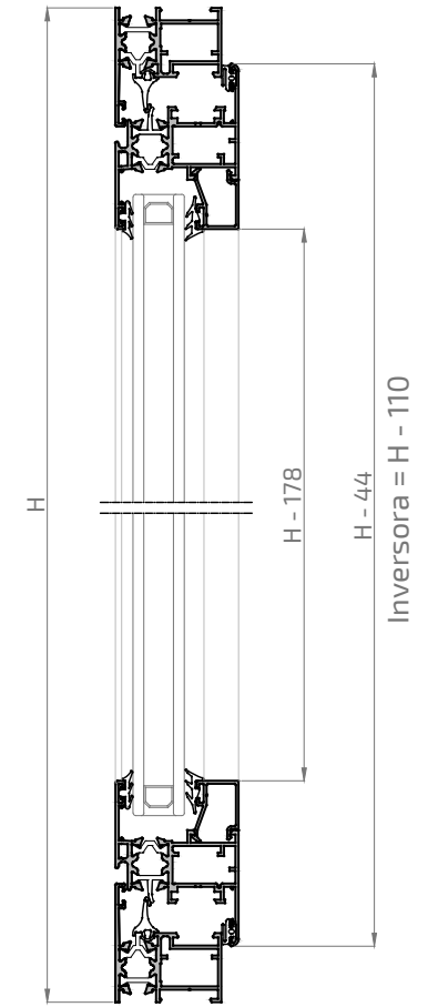
Sección B-B'
