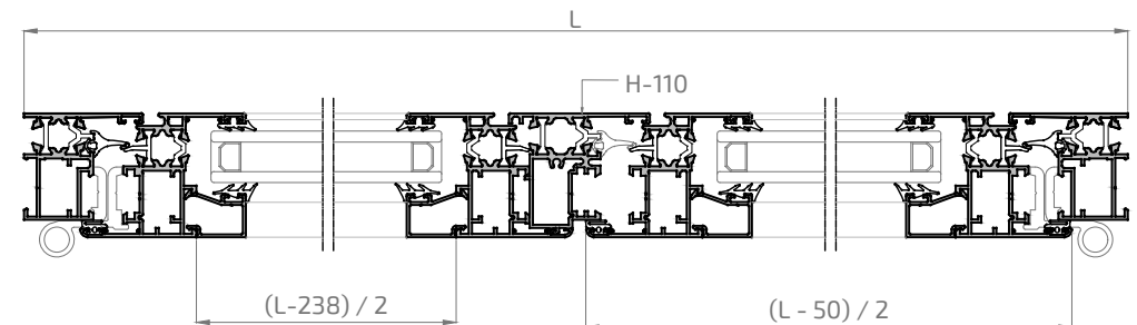
Sección A-A'
