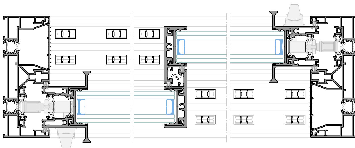
Sección A-A'
