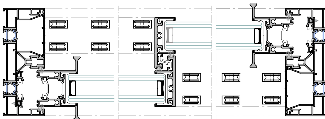
Sección A-A'
