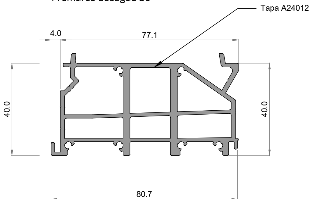
20994 Premarco desagüe 80
