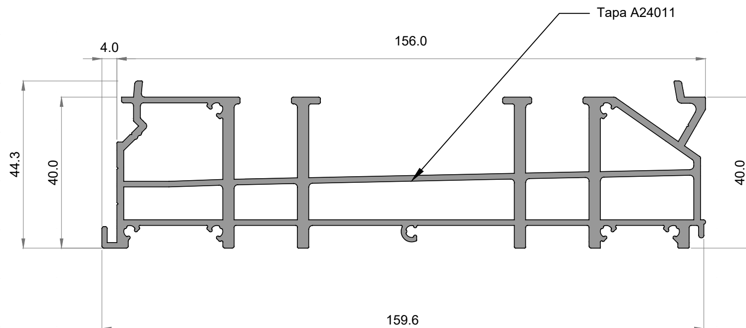
20994 Premarco desagüe 160
