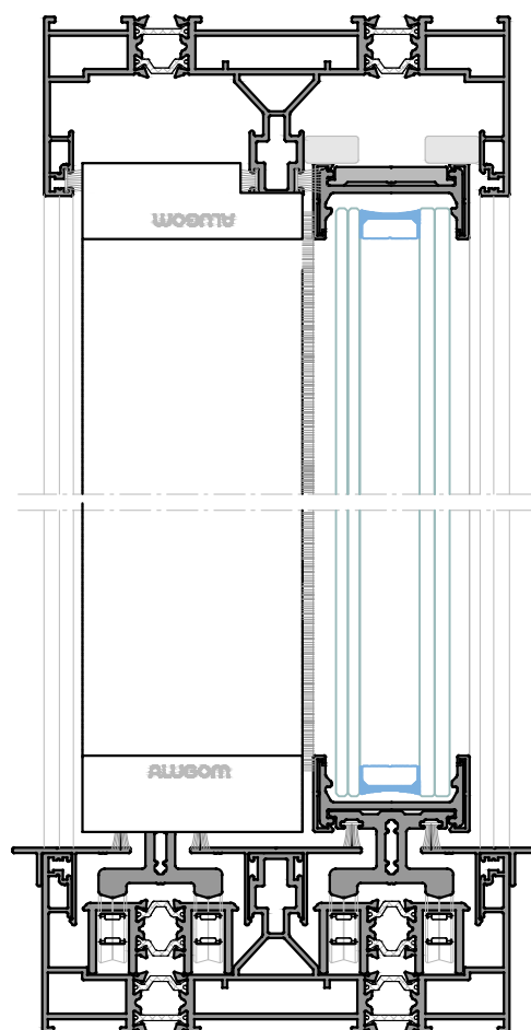
Sección B-B'
