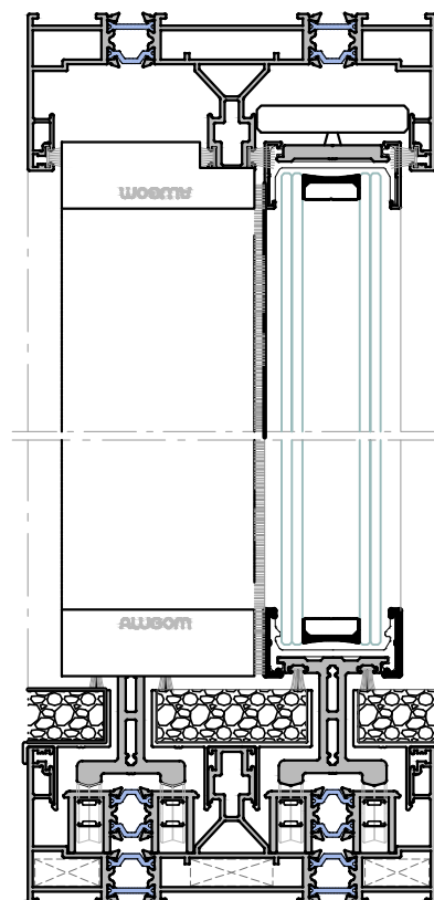
Sección B-B'
