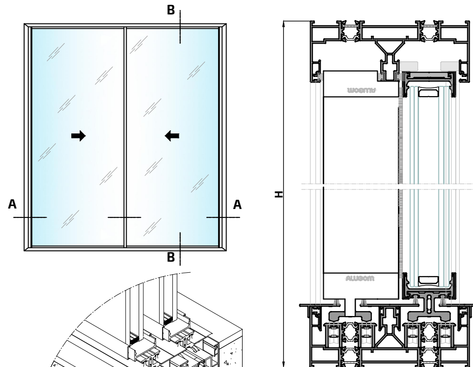
Sección B-B'
