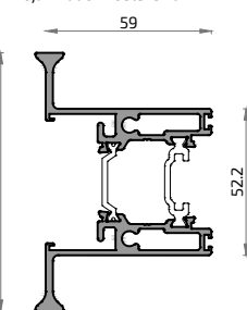
16261L Hoja Tirador Doble Ibiza
