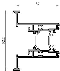
18440L Hoja Tirador Doble Cerradura Ibiza
