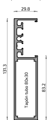
16837 Hoja Central 4 Hojas Ibiza
