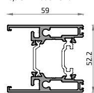
18193L Hoja Sin Tirador Ibiza
