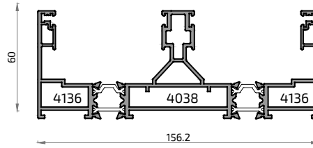
10966 Tapa Cobertura Cercos Ibiza
