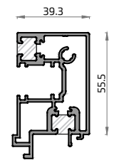
18175A Esquinero Ibiza
