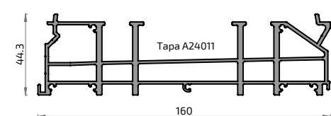
20994 Premarco Desagüe 160
