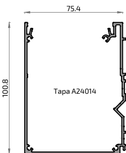
20978 Canalón 100 I-Cover
