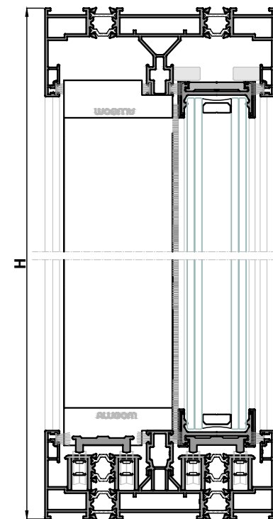
Sección B-B'
