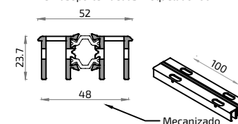
10969MT Perfil Soporte Ruedas Troquelado 100 mm
