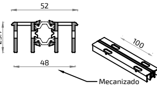
10969MT Perfil Soporte Ruedas Troquelado 100 mm
