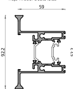
16261L Hoja Tirador Doble Ibiza
