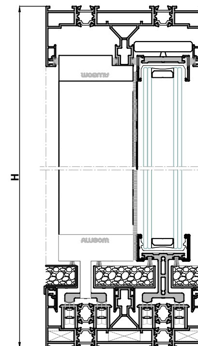
Sección B-B'
