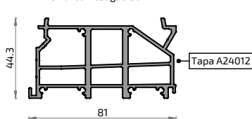
20993 Premarco Desagüe 80
