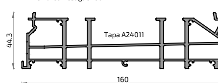
20994 Premarco Desagüe 160
