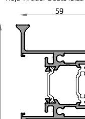
16261L Hoja Tirador Doble Ibiza
