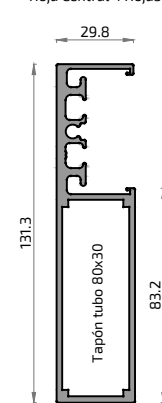
20993 Premarco Desagüe 80
