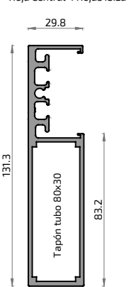
16837 Hoja Central 4 Hojas Ibiza
