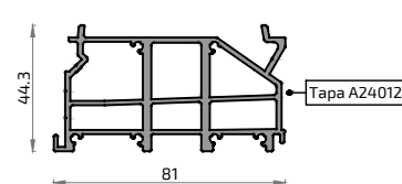
20993 Premarco Desagüe 80
