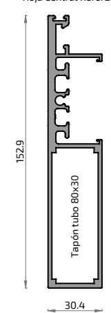
16838 Hoja Central Reforzada Ibiza
