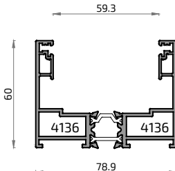
18193L Hoja Sin Tirador Ibiza
