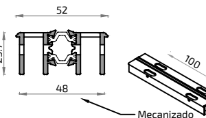
10969MT Perfil Soporte Ruedas Troquelado 100 mm
