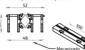
10969MT Perfil Soporte Ruedas Troquelado 100 mm
