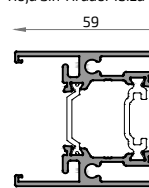
18193L Hoja Sin Tirador Ibiza
