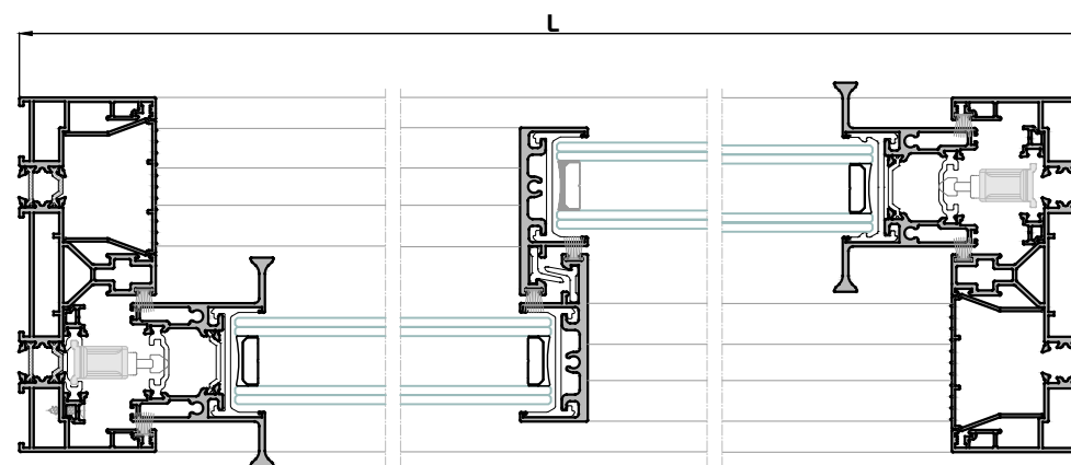
Sección A-A'
