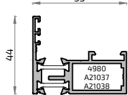
20206M Hoja cruce minimalista Matra 135
