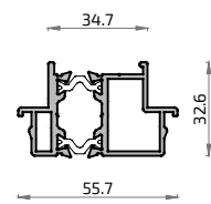
8680M Acople 4 Hojas Matra 135 RPT
