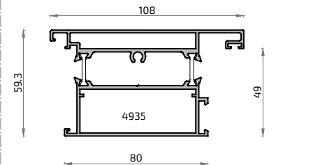
8971M 1171M Pilastra Monocarril Matra 135 RPT
