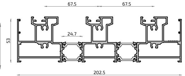
21130M Cercos simétrico 3 carriles
