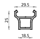
783 6695 Base Refuerzo Postizo Hoja
