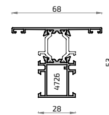
8865L Pilastra 28 mm Matra 135 RPT
