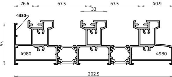
8682M Cercos 3 Carriles Matra 135 RPT
