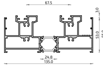
20206M Hoja cruce minimalista Matra 135
