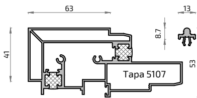
16104 Esquinero Hoja Matra 135 RPT
