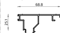
8973 Tapa Exterior Cercos Monocarril Matra 135 RPT
