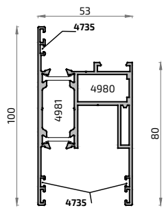
8673M 1163M Hoja Perimetral Matra 135 RPT
