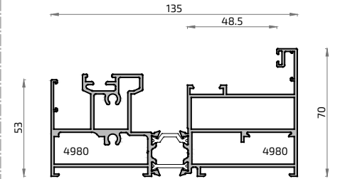
8974M Cercos Monocarril Matra 135 RPT
