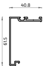
8676 1166 Acople Central Hoja Matra 135 RPT
