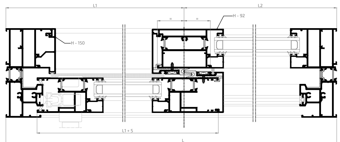
Sección A-A'
