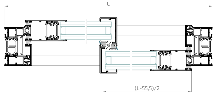
Sección A-A'
