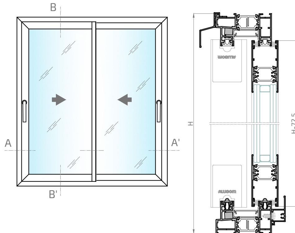
Sección B-B'
