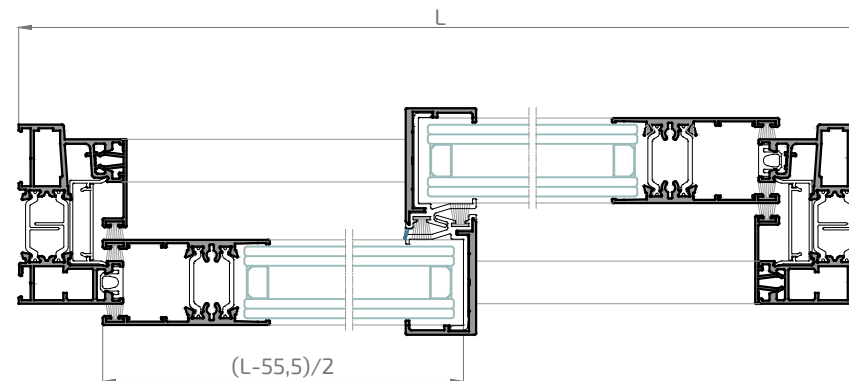
Sección A-A'
