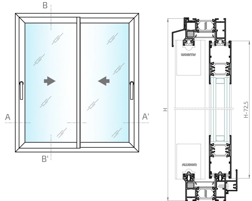
Sección B-B'
