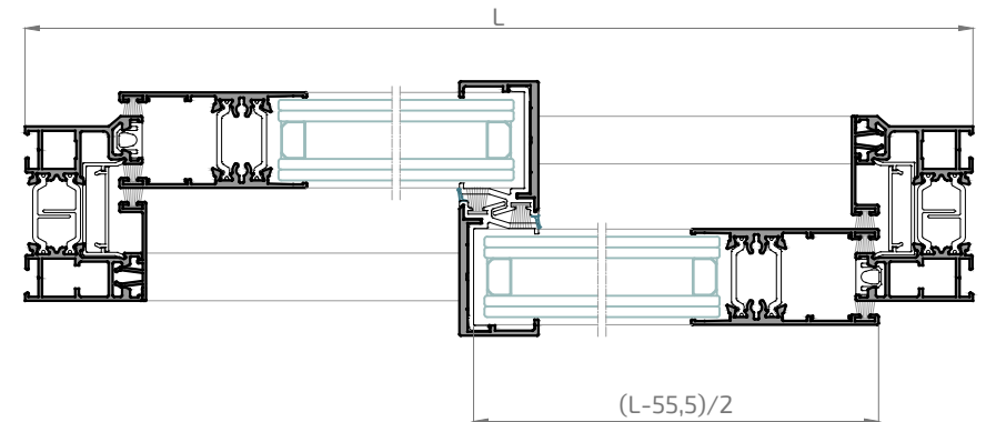
Sección A-A'
