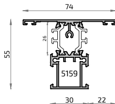
16690L Pilastra 30 alg 55
