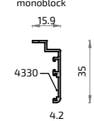
8832 Solapa inferior 30 mm para monoblock
