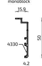
8630 Solapa inferior 45 mm para monoblock
