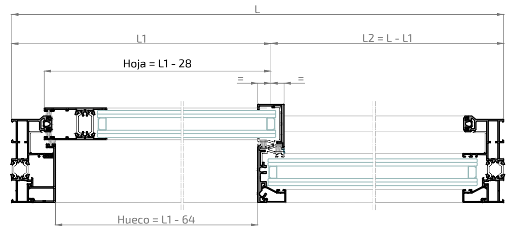
Sección A-A'
