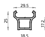
783 6695 Base refuerzo postizo hoja
