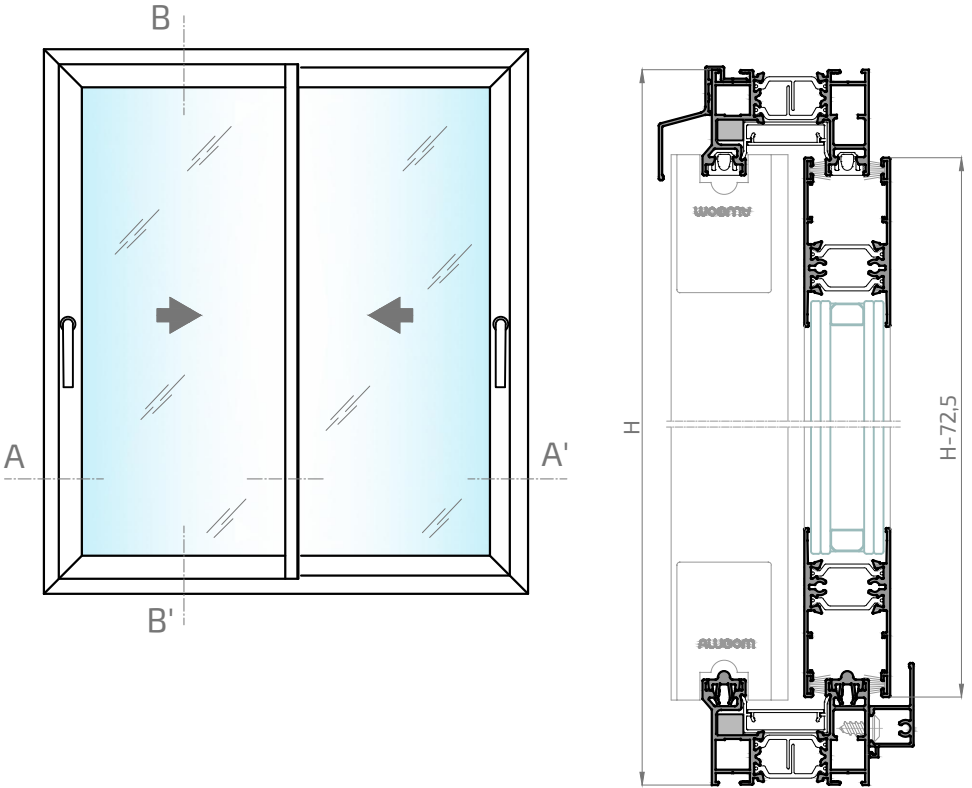
Sección B-B'
