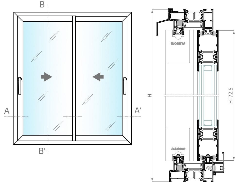
Sección B-B'
