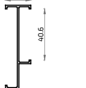
583 6653 Unión de cercos reductor
