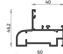
8593 NO STOCK Cercos Fijo Registro 60 mm S-350E
