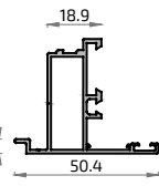
20140 Perfil Inversor
