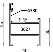
311 3586 Cercos Portada 36mm S-350E
