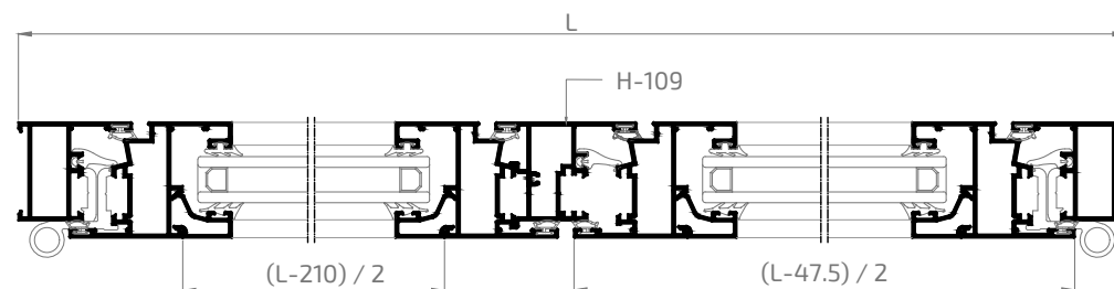
Sección A-A'
