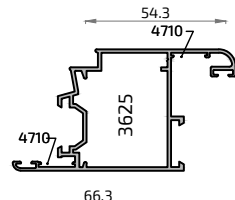
20140 Perfil Inversor
