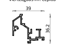
369 3548 Solapa 50 mm
