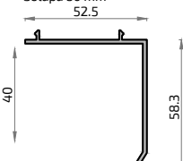
369 3548 Solapa 50 mm
