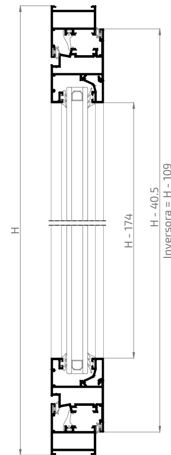
Sección B-B'
