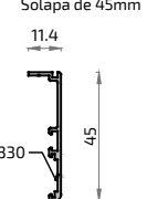
8629 Solapa de 45mm
