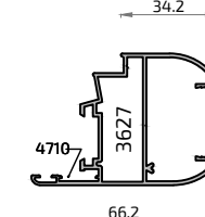
20143 Pilastra Reforzada Ancha
