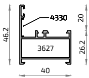
300 3575 Cercos de 40 mm S-350E
