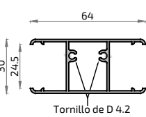
8296 Divisor Hoja s/junq. Dobl. Crist. S-350E
