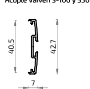
142 2579 Acople Vaivén S-100 y 350
