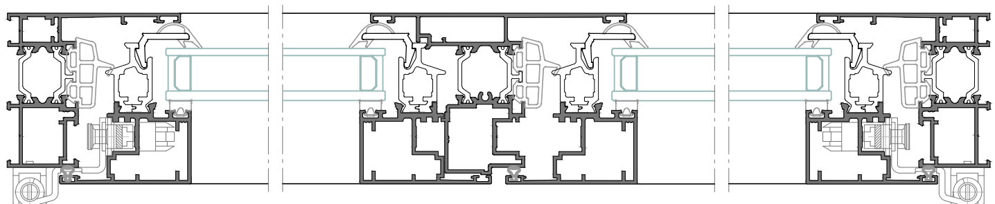
Sección A-A'
