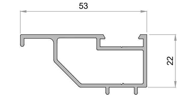
717 1207 Acople junquillo ALG 65 HS
