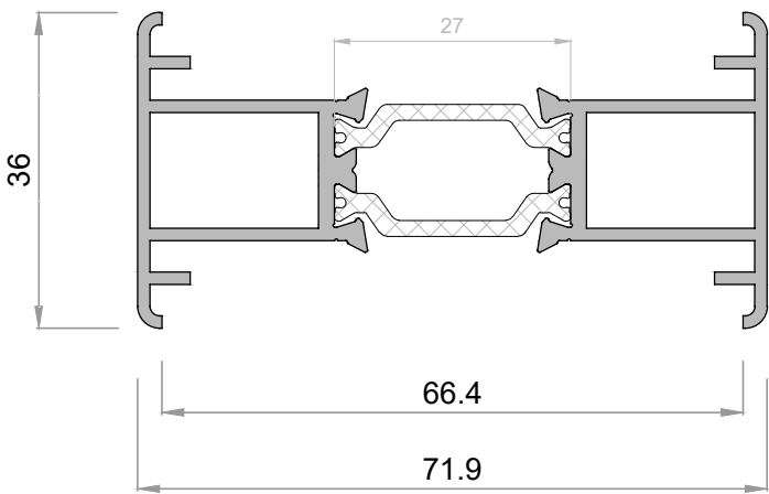
8482L Unión de cercos alg 65
