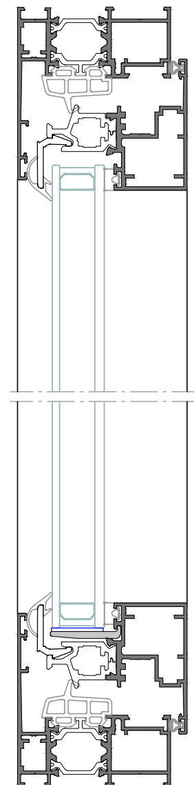
Sección B-B'
