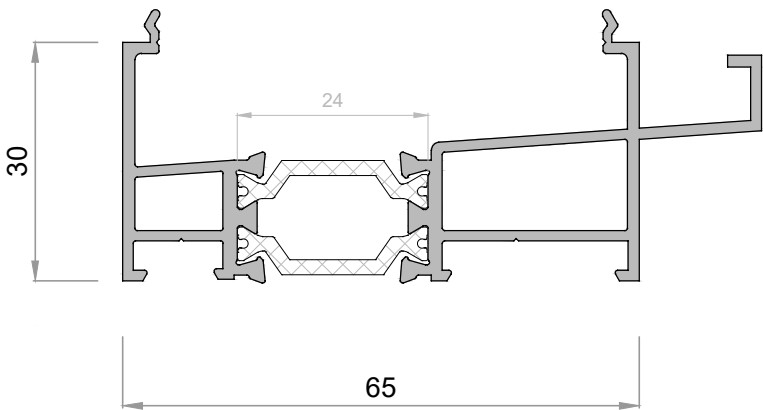
16319L NO STOCK Condensación 65 mm alg 65
