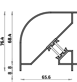
10006M Esquinero 90° Curvo
