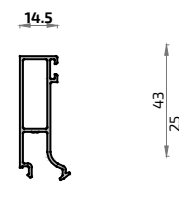
20334 Junquillo largo 14,5 mm
