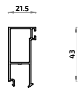
20318 Junquillo largo 21,5 mm
