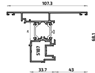
16781L Acople inversora alg 65 HS C16
