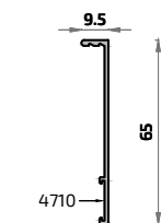
16323 Solapa clip 65mm
