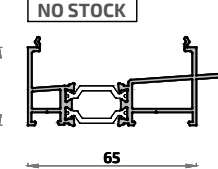
16319L Condensación 65 mm alg 65
