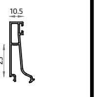
21087 Junquillo largo 10,5 mm
