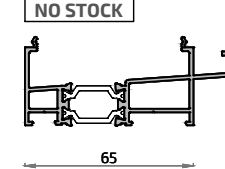
16319L Condensación 65 mm ALG 65
