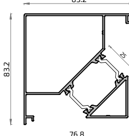
18215L Esquinero 90° Recto
