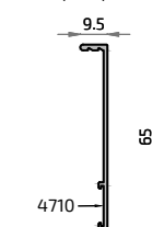
16323 Solapa Clip 65 mm
