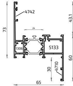
8190L NO STOCK Cercos Solape 30 mm ALG 65 HS
