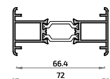
8482L Unión de Cercos ALG 65
