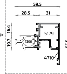
20354L Hoja ALG 65 Óptima HS C16
