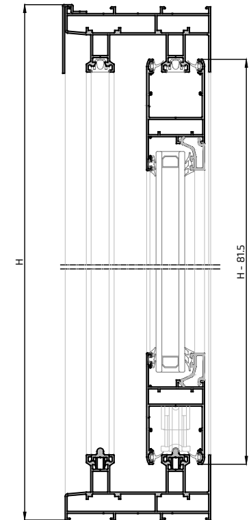
Sección B-B'
