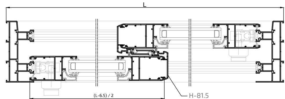
Sección A-A'
