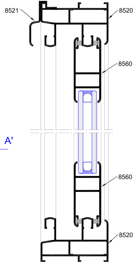
Seccion B-B'
