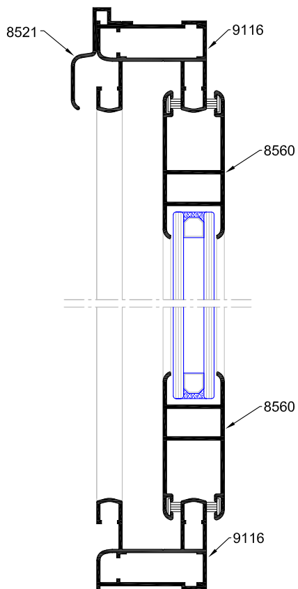
Seccion B-B'
