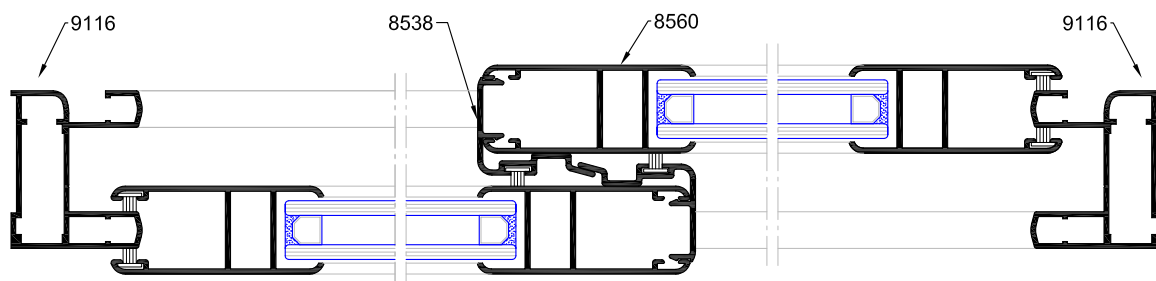
Seccion A-A'
