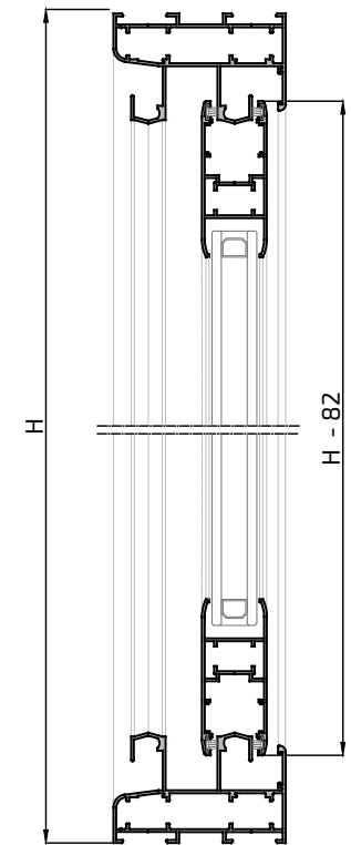
Sección B-B'
