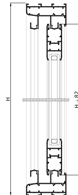
Sección B-B'
