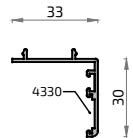
1434 327 Solapa Clip 30 mm
