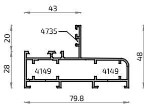
8598 Cercos Fijo 80 mm Silver 76
