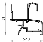
21003 Carril Suplementario Silver 76
