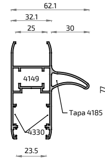
8580 Hoja con Tirador Silver 76
