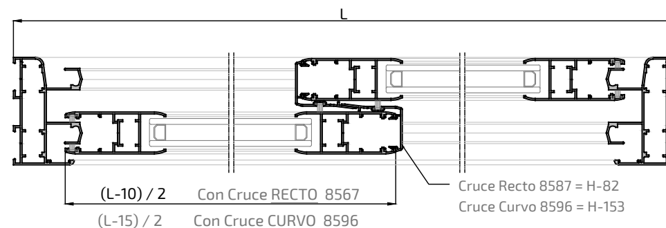
Sección A-A'
