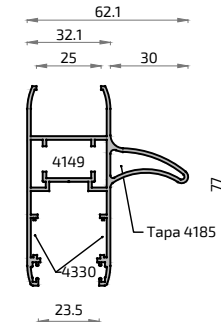
8580 Hoja con Tirador Silver 76
