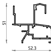
21003 Carril Suplementario Silver 76
