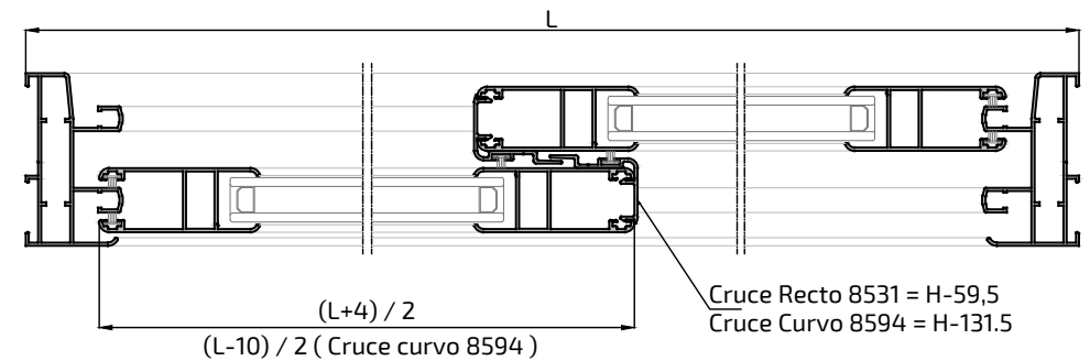
Sección A-A'
