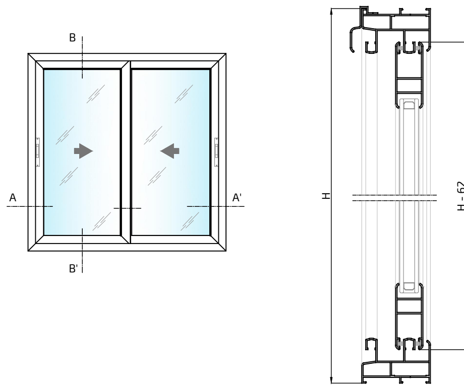
Sección B-B'
