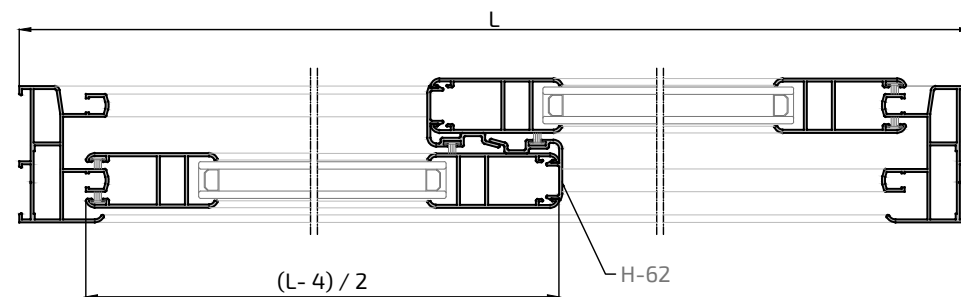
Sección A-A'
