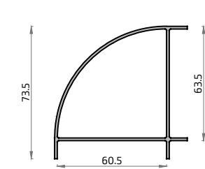
614 6101 Esquinero 60 mm
