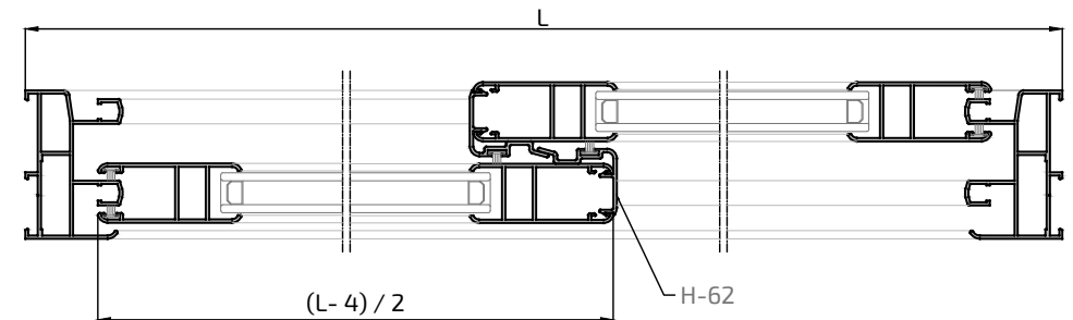
Sección A-A'
