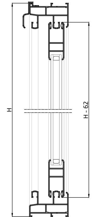
Sección B-B'
