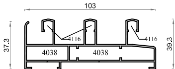
8519 Cercos Perimetral 3 Carriles Silver 60
