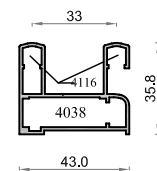
9116 NO STOCK Cercos Perimetral Reducido de 43mm Silver 60
