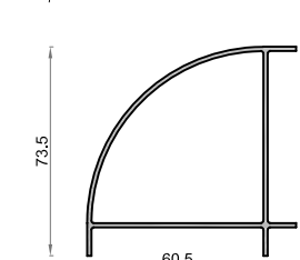
614 6101 Esquinero 60 mm
