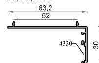
461 2233 Solapa Clip 30 mm
