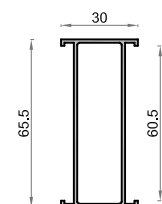
871 3061 Solapa Clip 50 mm
