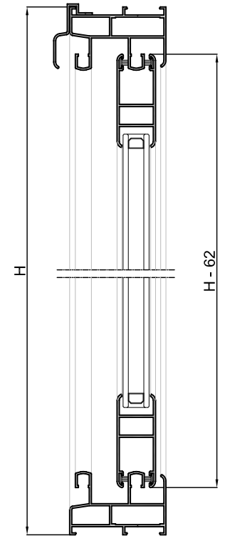
Sección B-B'
