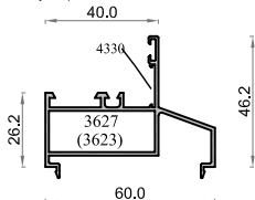
507 6611 Esquinero Regul. Tubo 60 mm
