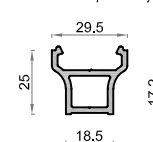
783 6695 Base refuerzo postizo hoja
