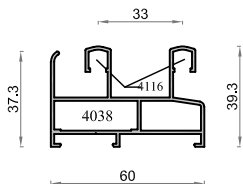
8520 Cercos Perimetral Silver 60
