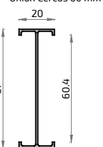
613 6110 Unión Cercos 60 mm
