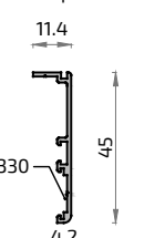
8629 Solapa de 45mm
