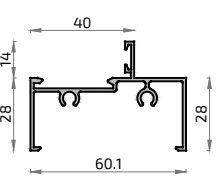
506 6612 Esquinero 60x40 mm.
