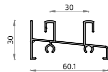
451 2227 Hoja Ruedas Dobl. Cristal 52 mm S-400E
