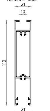
448 2238 Zócalo Cristal Sencillo 110 mm S-400E
