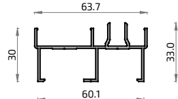
470 2251 Hoja Lateral 55mm Dobl. Cr. S-400E
