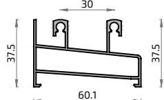
447 2223 Hoja de Ruedas 52 mm S-400E
