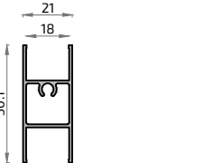
464 2239 Divisor Hoja Dobl. Cristal S-400E
