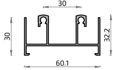
449 2225 Hoja Lateral Dobl. Cr. 53 mm S-400E
