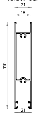
452 2228 Zócalo Dobl. Cristal 110 mm S-400E
