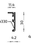
281 1140 Solapa de 30mm
