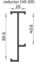
583 6653 Unión de cercos reductor (40-60)
