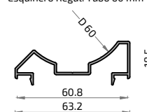
507 6611 Esquinero Regul. Tubo 60 mm
