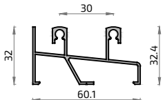
445 2221 Hoja Lateral 53mm S-400E
