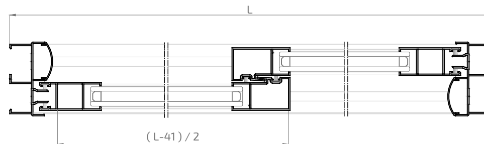
Sección A-A'
