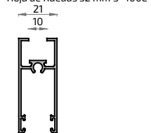
464 2239 Divisor Hoja Dobl. Cristal S-400E
