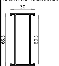
511 6622 Unión Cercos Tubul. 60 mm
