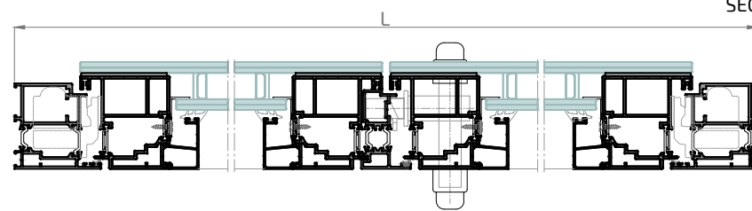
SECCIÓN A-A'
