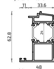
18394L Suplemento Inversor Marco Apertura Exterior
