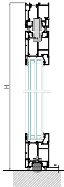
SECCIÓN B-B'
