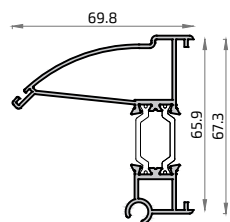
18897L Esquinero Regulable Hembra ALG 65
