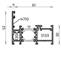
16332L Cerro 30 mm
