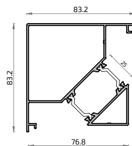
18215L Esquinero 90°
