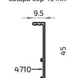
16322 Solapa Clip 45 mm
