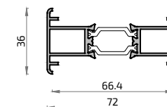
8482L Unión de Cercos 65 mm
