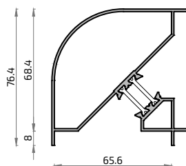
10006M Esquinero Curvo
