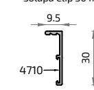
16321 Solapa Clip 30 mm
