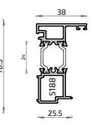
17279L Acople Inversora ALG PUERTA
