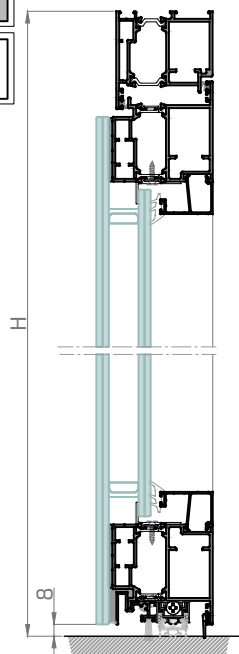
SECCIÓN B-B'
