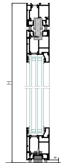
SECCIÓN B-B'
