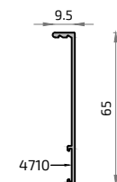
16323 Solapa Clip 65 mm
