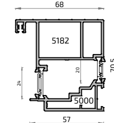
18152L Hoja Apertura Externa ALG GLASS
