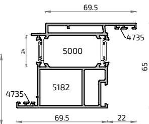
17187L Hoja ALG PUERTA Apert. Interna
