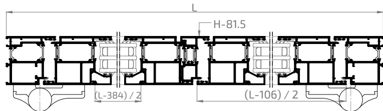
SECCIÓN A-A'
