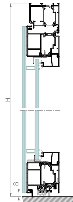
SECCIÓN B-B'
