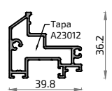
20338 Perfil Suelo Puerta
