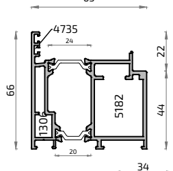
17186L Cerro ALG PUERTA 65
