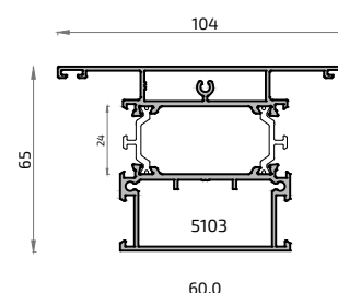
18181L Pilastra 60 mm ALG 65
