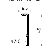
16322 Solapa Clip 45 mm
