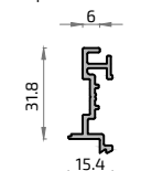
20822 Batiente Vaivén
