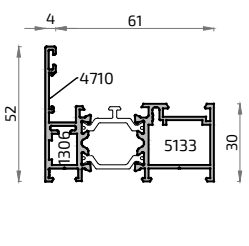
16332L Cercos 30 mm
