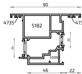
17277L Hoja Apertura Externa ALG PUERTA
