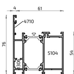
16300L Cercos 54 mm
