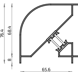
10006M Esquinero Curvo
