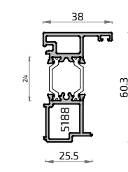
17279L Acople Inversora ALG PUERTA
