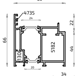
17186L Cercos ALG PUERTA 65
