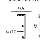
16321 Solapa Clip 30 mm
