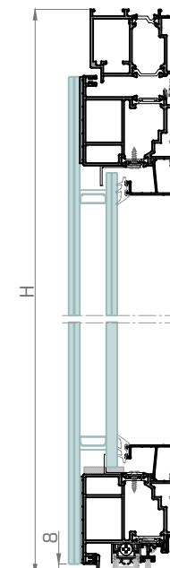
SECCIÓN B-B'
