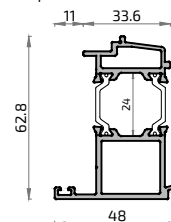
18394L Suplemento Inversor Marco Apertura Exterior
