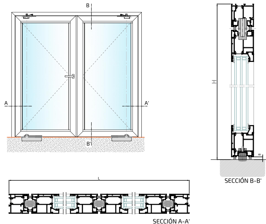
PUERTA 2 Hoja Practicables VAIVÉN
