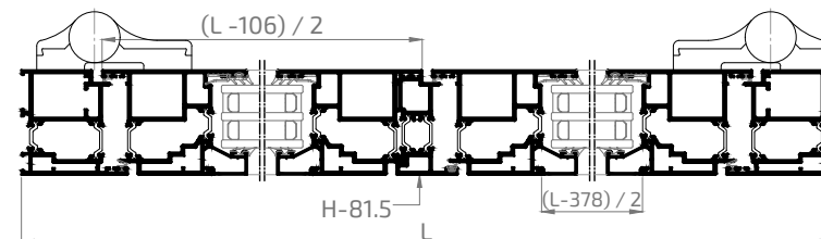
SECCIÓN A-A'
