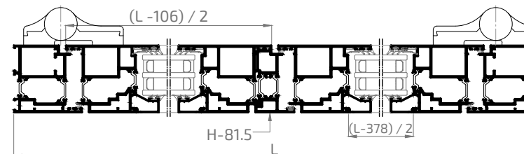
SECCIÓN A-A'
