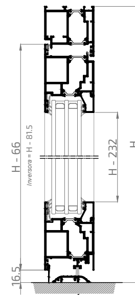
SECCIÓN B-B'
