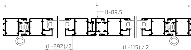
SECCIÓN A-A'
