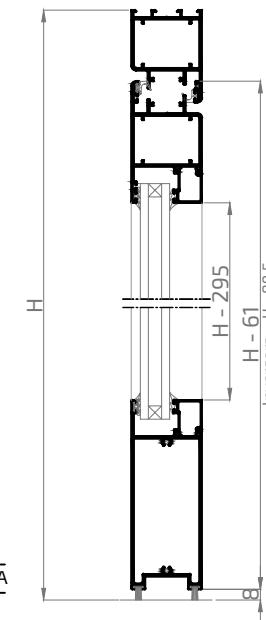
SECCIÓN B-B'
