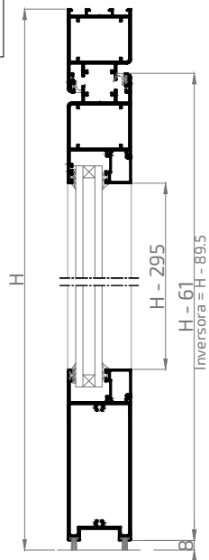
SECCIÓN B-B'
