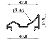
148 2593 Esquinero Regul. Tubo 40
