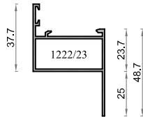
134 2542 Cercos con Solapa S-100
