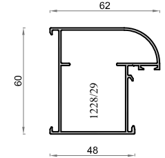
180 2591 Cercos Escaparate 48 mm S-100
