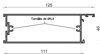
123 2507 Cercos Zócalo 111 mm S-100
