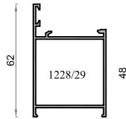
115 2548 Cercos 48 mm S-100
