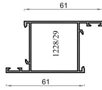
116 2550 Hoja Lisa Portada S-100
