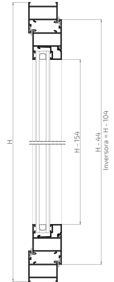
Sección B-B'
