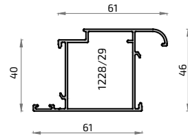
147 2594 Hoja Balconera Curva S-100
