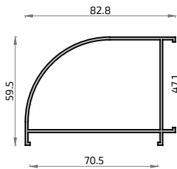
506 6612 Esquinero 60x40 mm
