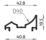
148 2593 Esquinero Regul. Tubo 40
