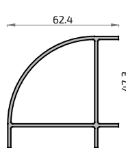
630 6102 Esquinero Redondo 40 mm
