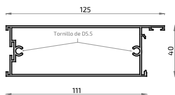
123 2507 Cerco Zócalo 111 mm S-100
