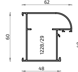
180 2591 Cerco Escaparaté 48 mm S-100
