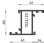
101 2544 Hoja Lisa Ventana S-100
