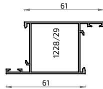
116 2550 Hoja Lisa Portada S-100
