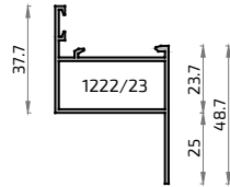
134 2542 Cerco con Solapa S-100
