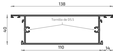
120 2508 Manguetón Central 110 mm S-100
