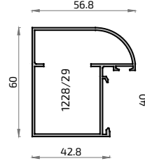
126 2526 Cerco Escaparaté 43 mm S-100
