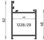
115 2548 Cerco 48 mm S-100
