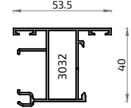
137 2533 Acople Inversora S-100
