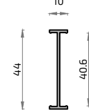
646 6144 Unión Cercos 40 mm
