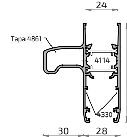
10007M Hoja Reforzada 74,5 mm Silver 65RPT
