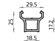
783 6695 Base refuerzo postizo hoja
