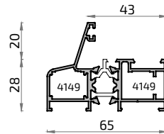
8897M Cercos Fijo 65 mm Silver 65RPT
