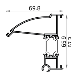
18897L Esquinero regulable hembra 65
