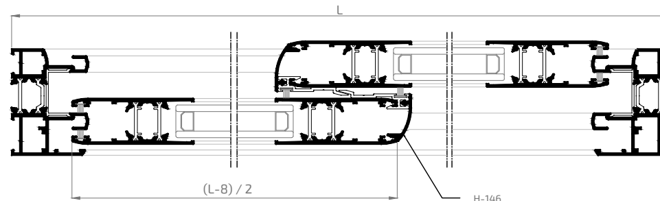
Sección A-A'
